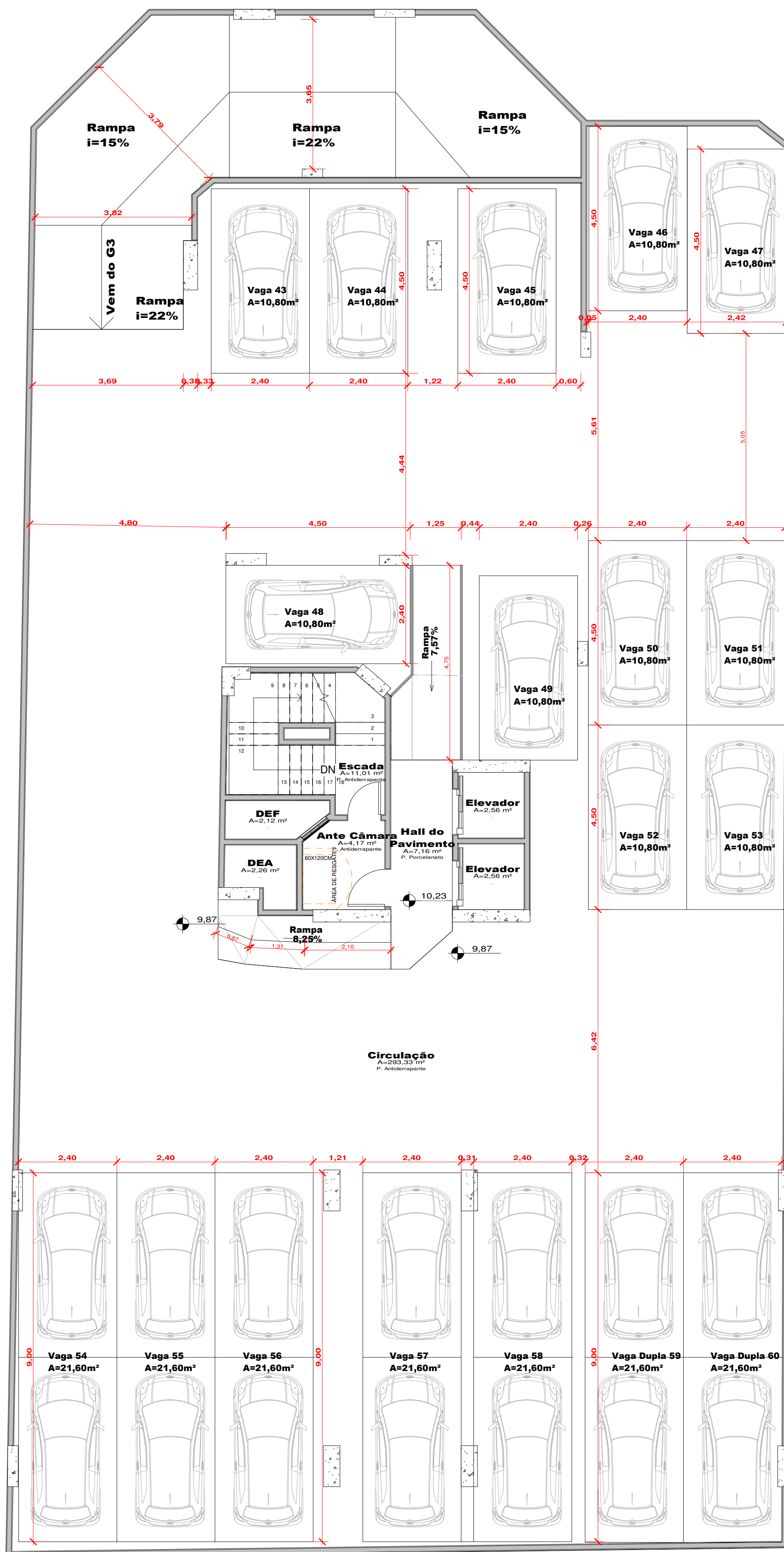
1 Pavto Garagem 04 1 : 75
